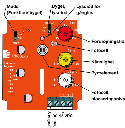
Kretskort i närvarodetektor PD-231
