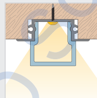
Montage mit 180° Abdeckung z.B. als Schrank- unterbau mit Schraube mounting the 180° cover e.g. as under cabinet with screws
