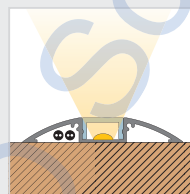
Montage auf Böden zur Beleuchtung mit integrierter Kabelführung mounting into floors for illumination with integrated cable duct
