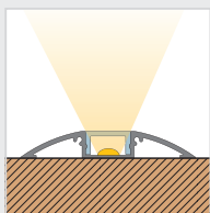
Montage auf Fußböden mounting on floors
