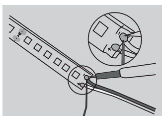
Ved lodding av stripen skal loddetemperaturen holde maks 300 °C. Følg polariteten nøye.
