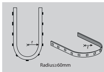
LED stripen skal aldri bøyes mer enn R = 60 mm.
