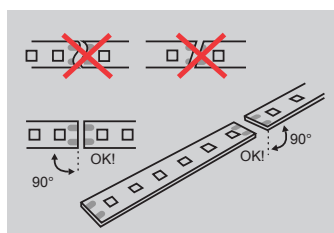
Klipp LED stripen med skarp saks og alltid i 90° som vist over!
